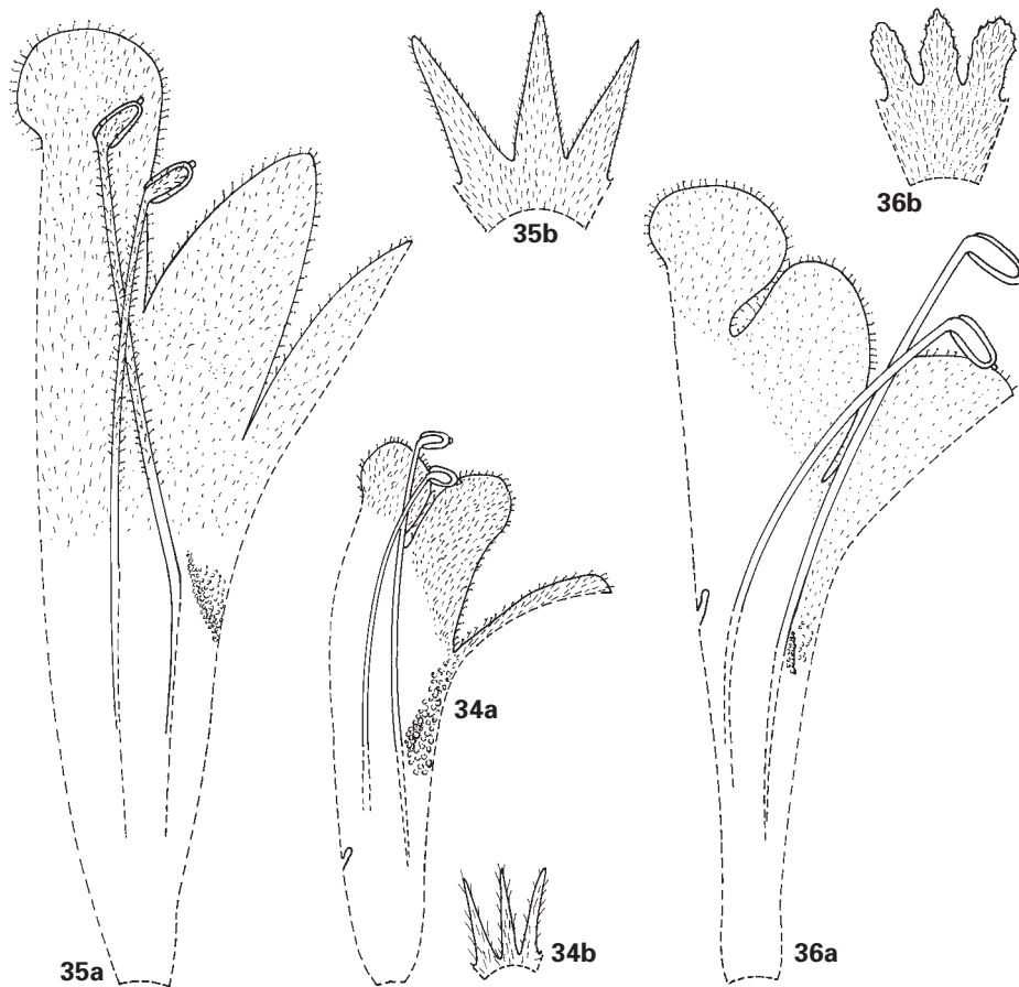
FIG. 15. Part of calyx and longitudinal section of corolla: 34a, b, A. scabriflora ; 35a, b, A. columneoides ; 36a, b, A. roseoflava . All \times 2 .
